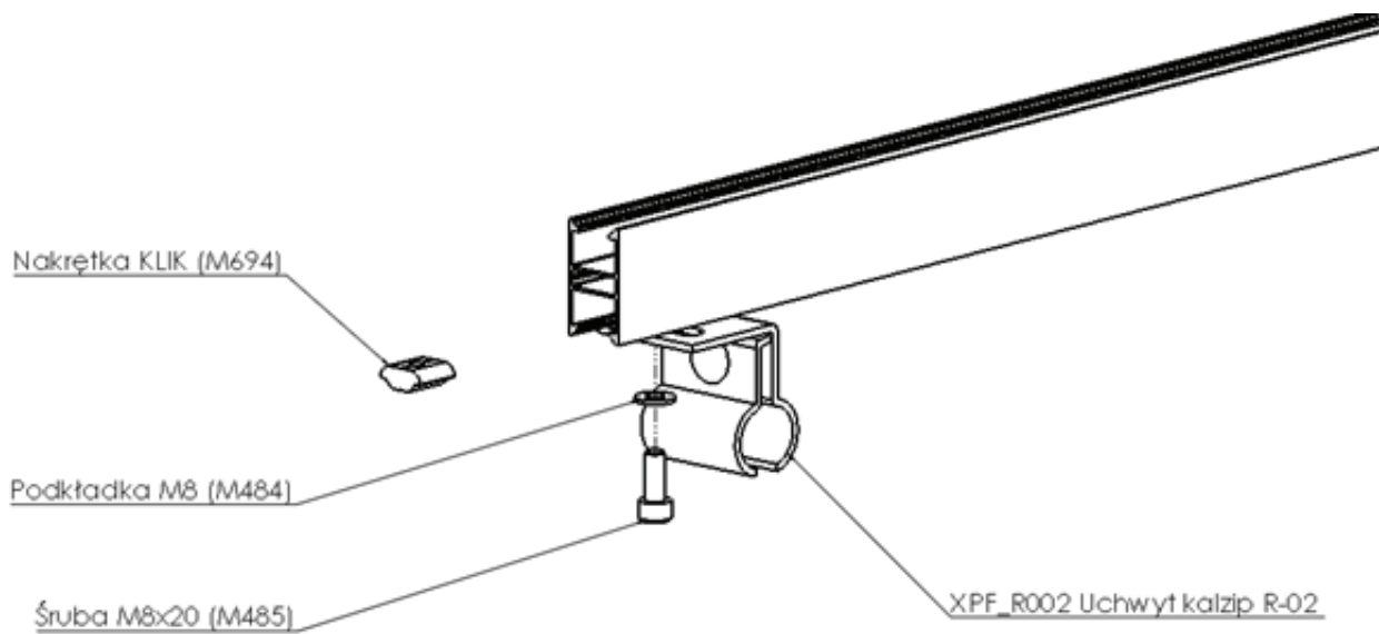
Rys.7. Połączenie szyny montażowej 26x47 z wspornikiem montażowym
