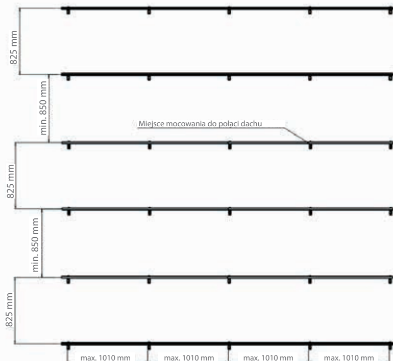
Rys.2. Ideowy plan rozmieszczenia szyn montażowych
