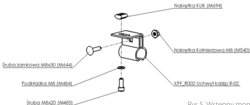
Rys.5. Wstępny montaż wsporników konstrukcyjnych systemu Corab
