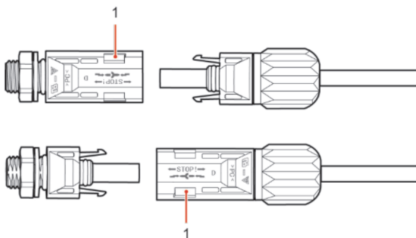
Rysunek 5-9 Podłączanie wejściowych kabli solarnych prądu stałego DC
