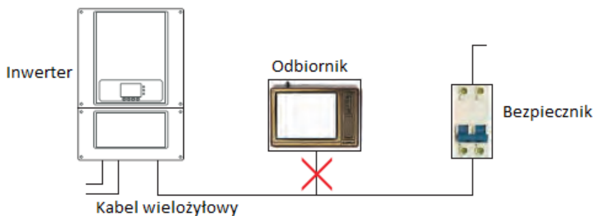
Rysunek 5-11 Nieprawidłowe podłączenie odbiorników elektrycznych
