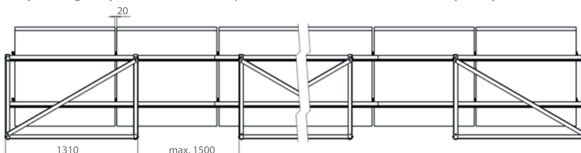
Rys.2 Ideowy plan konstrukcji
